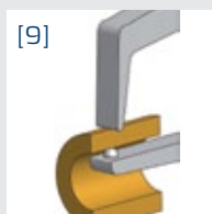
Cuchilla R 0,4 mm Bola Ø 1,5 mm
