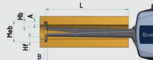
Meb Rango de medición A Profundidad de ranura B Anchura de ranura Hb Contacto móvil Hf Contacto fijo L Profundidad de medición
