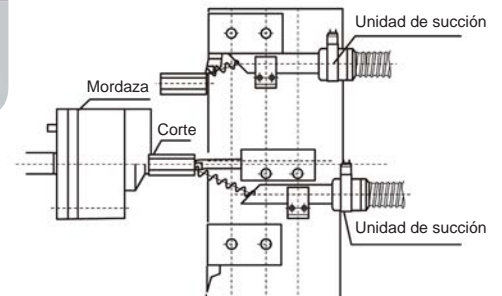
SUCCIÓN DE VIRUTAS DE CORTE CON UNIDAD FIJA
