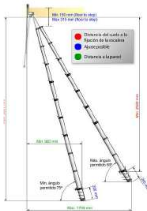
Medidas Loft 270
