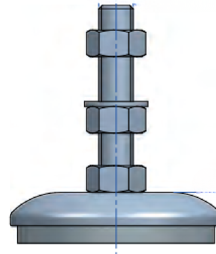
SOPORTE POLIURETANO OM REF. 144101 – M12 – 70 X 25 MM
