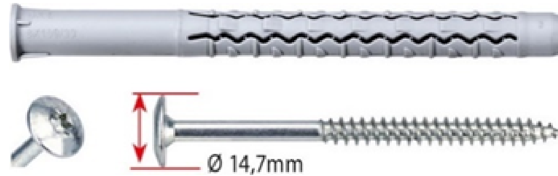
TACO GX-L NYLON VTF CON TORNILLO CABEZA GRANDE, TX30, PARAVENTANAS Y CERRAMIENTOS
